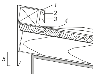
Skitse 11.3: Pulttagsrygning med træliste
