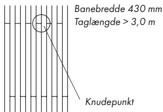
Skitse 2.2: Eksempel med pulit tag, taghældning 25°, baneinddeling med forskudt tværfals i forbandt (tværfals forskudt med en halv banelængde), stående dobbeltfals
