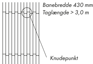
Skitse 2.3: Eksempel med pulit tag, taghældning 25°, baneinddeling med ca. 30 cm forskudt tværfals, stående dobbeltfals
