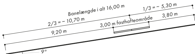
Skitse 2.1 til eksempel B: Pulttag, taghældning 9°, banelængde 16 m
