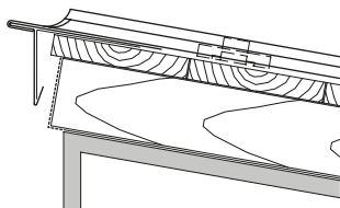
Skitse 11.4: Pulttagsrygning som tagfodsaflutning
