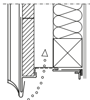
Skitse 17.1: Sokkelafslutning i niveau med ventilation
