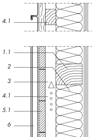
Skitse 14.1: Stående vinkelfalsbeklædning på underkonstruktion af træ
