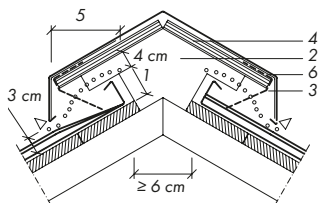
Skitse 11.2: Saddeltagrygning, taghældning > 25^\circ , udførselsvariant: lav udførelse med ventilationsspalter
